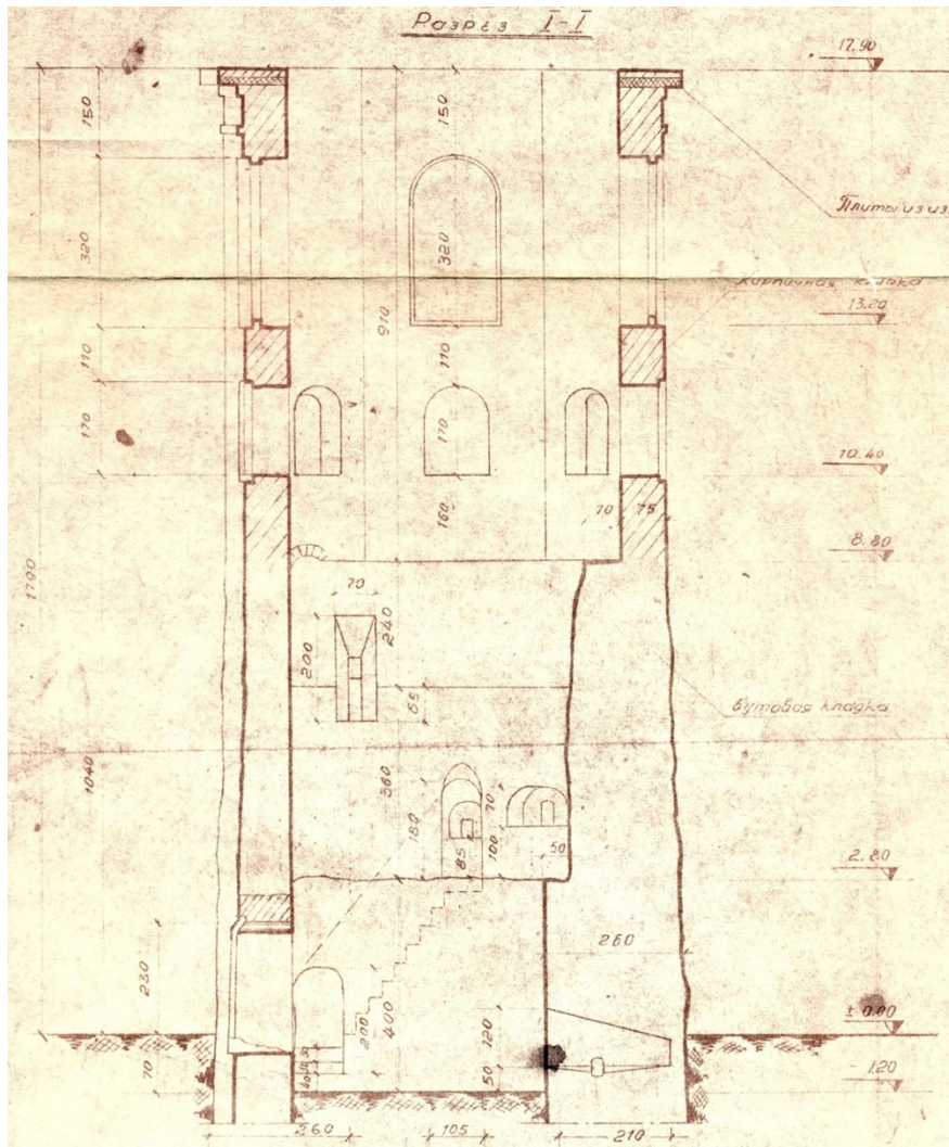
Raatitornin leikkaus mittauspiirustuksessa vuodelta 1949.
