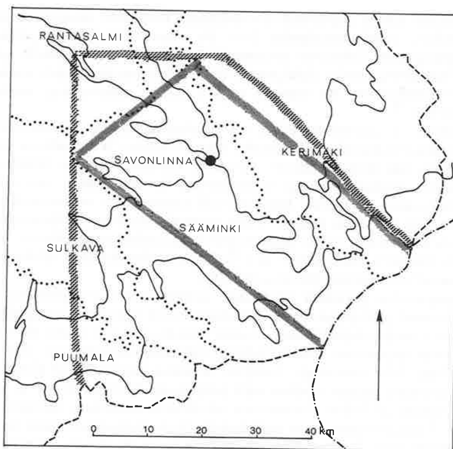
Kiista Savonlinnan ympäristön luovuttamisesta Venäjälle heinäkuun puolivälissä 1743. Ruotsin neuvottelijat olivat suostuvaisia antamaan noin puolta pienemmän alueen kuin venäläiset vähintään vaativat, sen jälkeen kun oli päästy yhteisymmärrykseen kahden peninkulman soveltamisesta. Suurin erimielisyys koski Sulkavaa ja Puumalaa, jotka Cedercreutz ja Nolcken halusivat säilyttää Ruotsilla. Kuvioon on merkitty pitäjänrajat pisteviivalla, Savon maakuntaraja katkoviivalla sekä valtakunnanraja piste-katkoviivalla.
