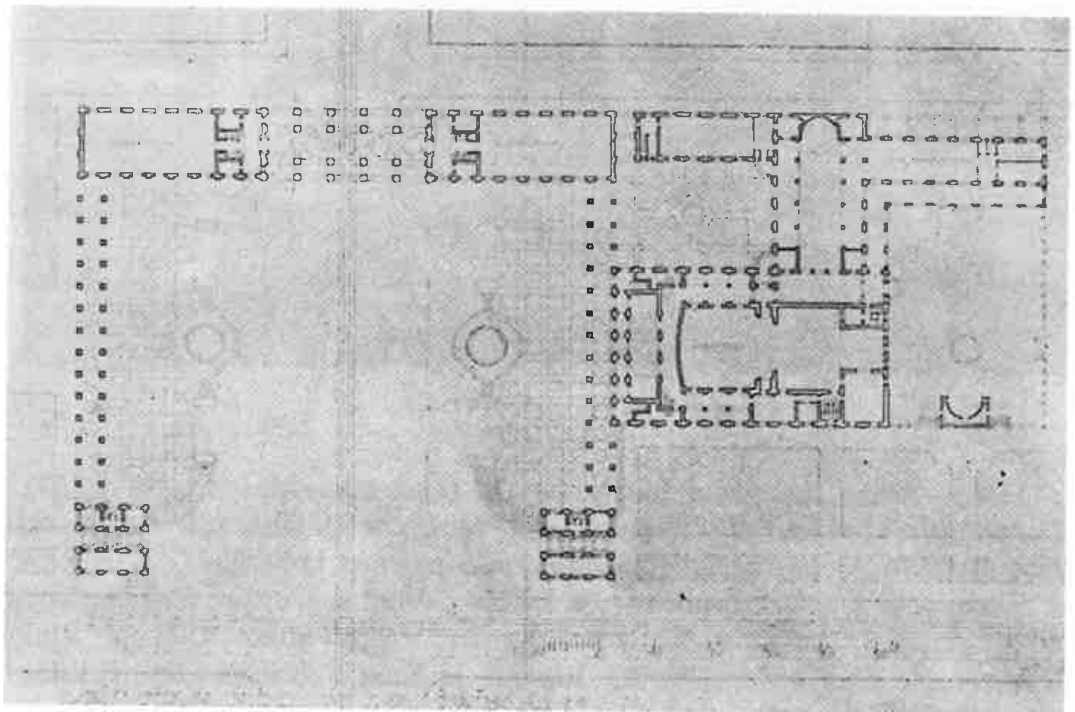
II palkinnon saaneiden W.G. Palmqvistin ja E. Sjöströmin ehdotuksen pohjapiirros
