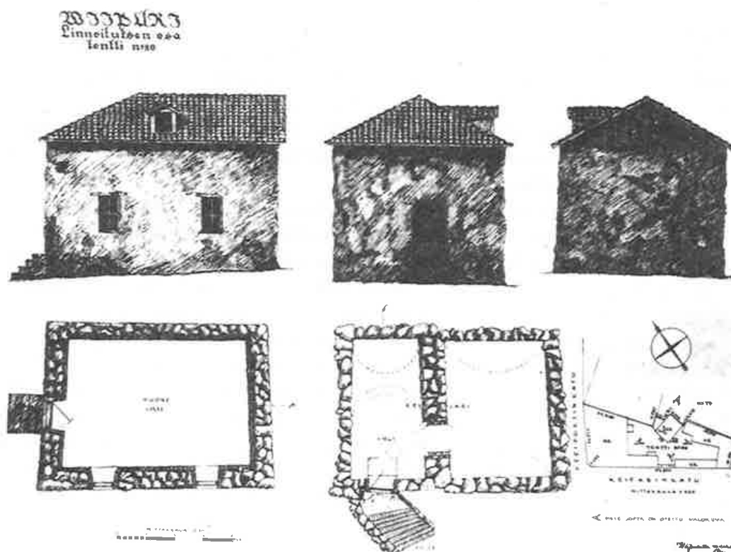
Luostarinkatu 8:n piharakennuksen mittauspiirustuksia 1935.
