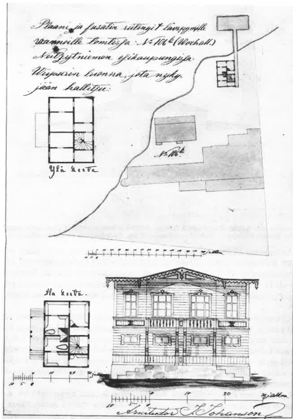
Kaupunginarkkitehti Johan Johansson laati 1860-luvulla Vauxhallia varten "plaani ja fasadin rii-tingit lämpymille wannille tomtissa N:o 106 b". Tyyli on jo koristeellisempaa kuin Bosinin aikana. Viipurin maistraatin arkisto, Savo-Karjalan maakunta-arkistossa.
