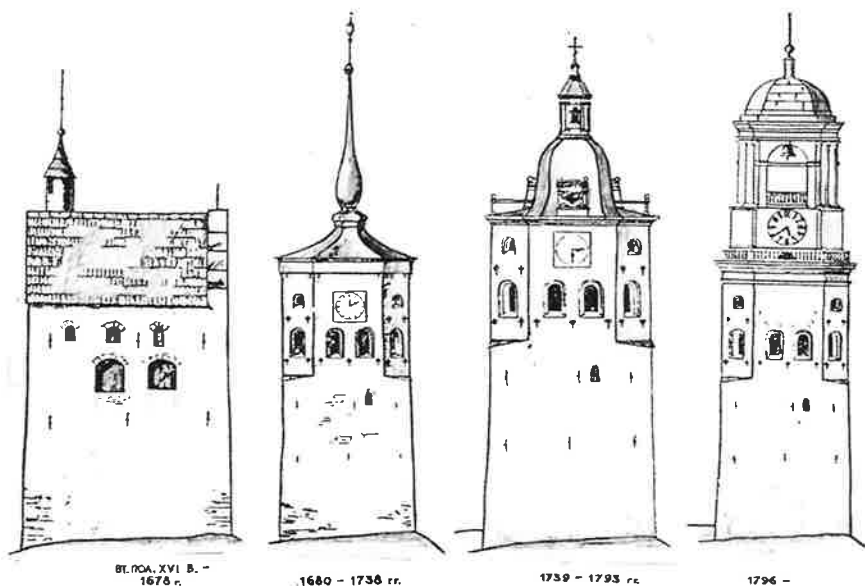
Kellotornin rakennusvaiheita esittävä piirrosarja lehdestä: Leningradin rakennukset ja arkkitehtuuri
